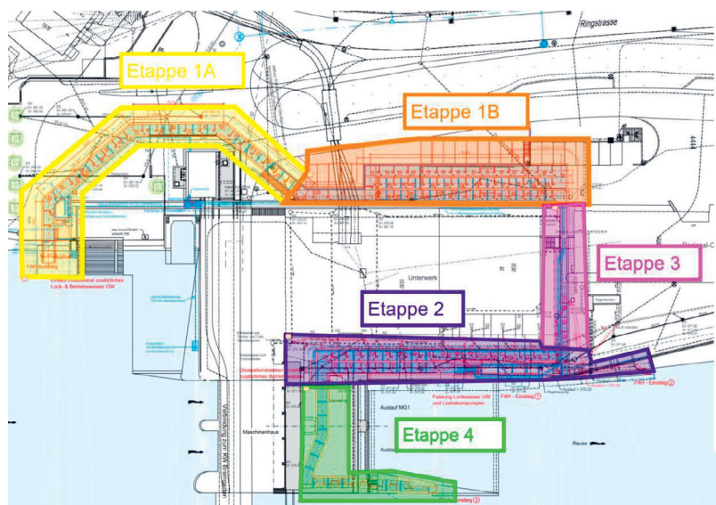
Bauetappen der Fischaufstiegshilfe
